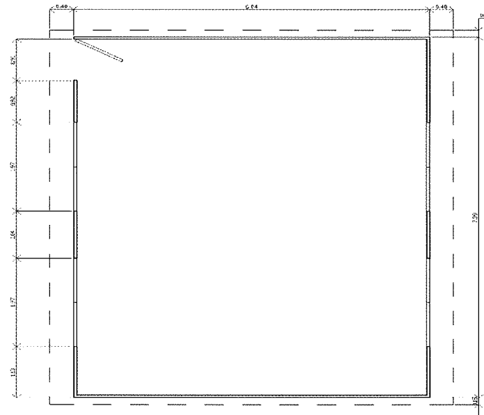
Aula Prefabricada Tipo, Planta Cotas: Metros esc 1:50
